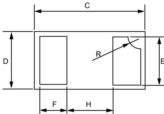
Bottom View(Optional)
